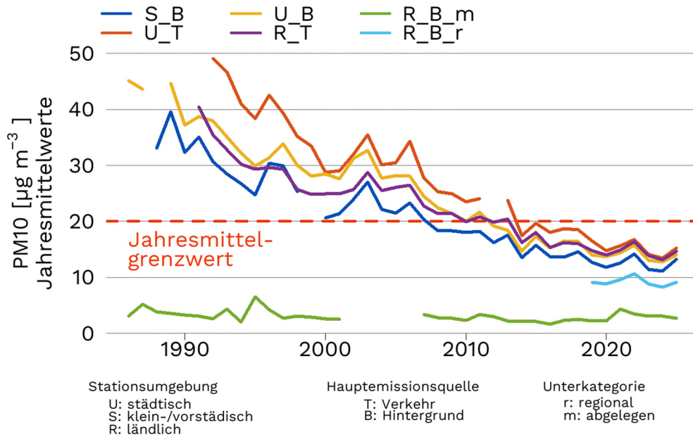
Entwicklung der PM10-Jahresmittelwerte 1986–2025 an verschiedenen Standorttypen des NABEL-Messnetzes [ \mu\text{g}/\text{m}^3 ]. Quelle: NABEL (BAFU und Empa).
