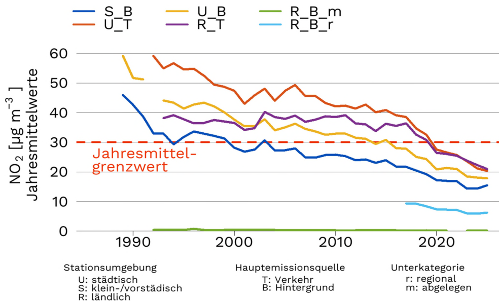
Entwicklung der \text{NO}_2 -Jahresmittelwerte 1988–2025 an verschiedenen Standorttypen des NABEL-Messnetzes [ \mu\text{g}/\text{m}^3 ]. Quelle: NABEL (BAFU und Empa).
