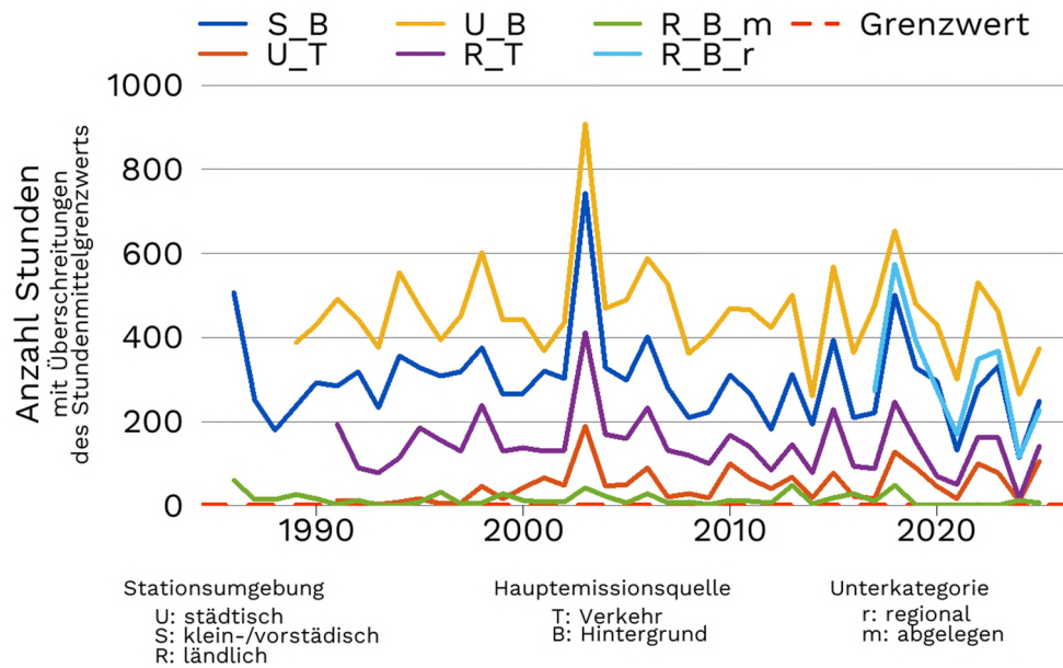
Immissionsentwicklung 1986-2025 an verschiedenen Standorttypen des NABEL-Messnetzes für Ozon [Anzahl Stunden mit Überschreitungen des Stundenmittelgrenzwertes]. Quelle: NABEL (BAFU und Empa).
