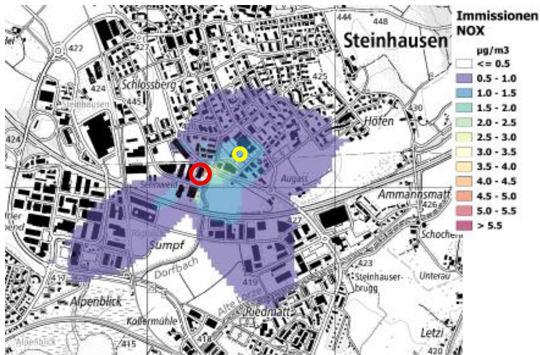
Abbildung 1: Modellierte Jahresmittelwerte von \text{NO}_x in \mu\text{g}/\text{m}^3 bei der geplanten Kaminbauhöhe von 35 m ab Baugrund. Der rote Kreis bezeichnet die Lage der Energiezentrale (2'679'287, 1'227'089) und der gelbe Kreis die Lage der Messstation in Steinhausen (2'679'508, 1'227'187). Quelle: Umweltbericht Energiezentrale Steinhausen. 1
