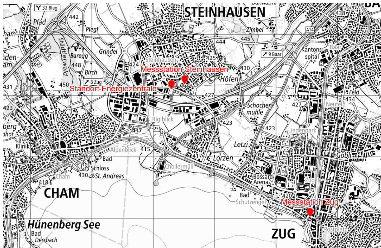
Abbildung 2: Standorte der Messstation in Steinhausen (2'679'508, 1'227'187) auf dem Areal der ehemaligen Crypto AG sowie der Referenz-Messstation in Zug (2'681'625, 1'224'641) am Postplatz. Eingezeichnet ist ebenfalls der Standort der Energiezentrale in Steinhausen.
